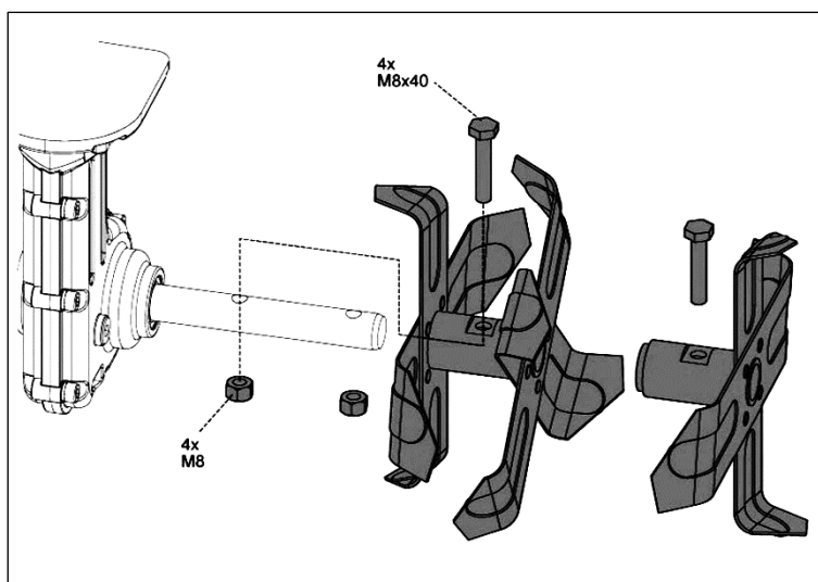
Рис.4 Установка фрез
