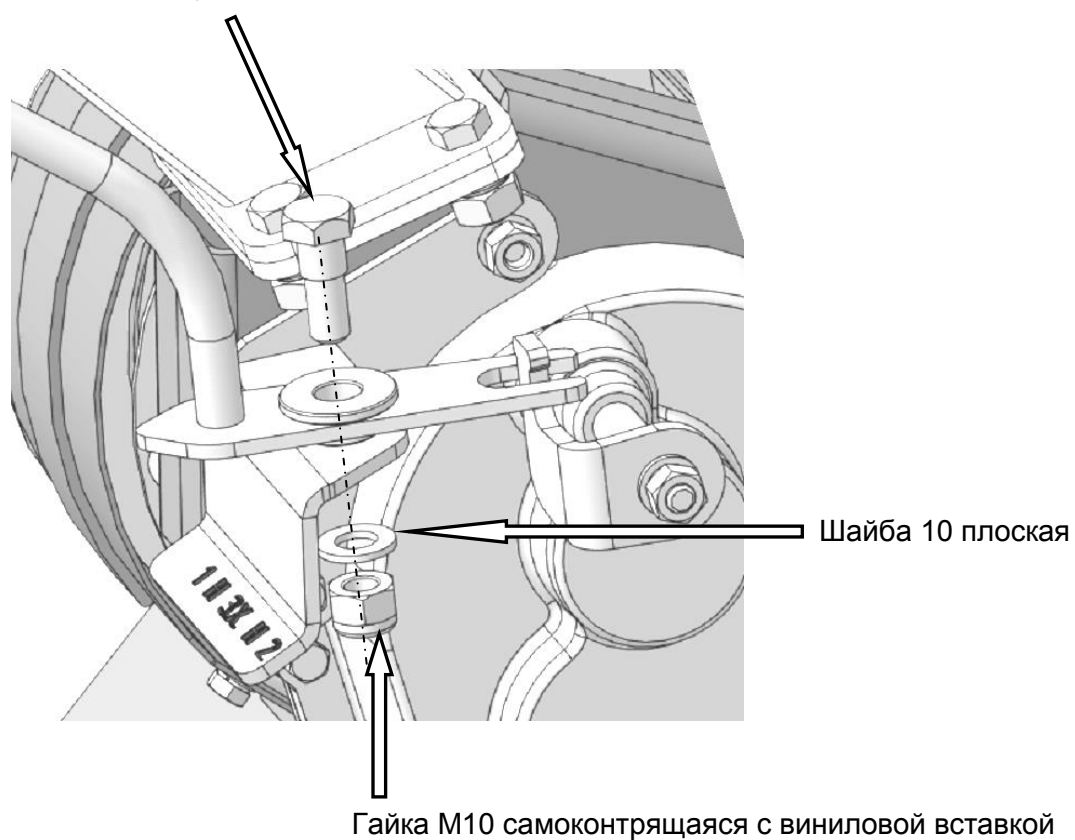
Рис.4. Схема сборки мотоблока с ручкой включения скоростей.
