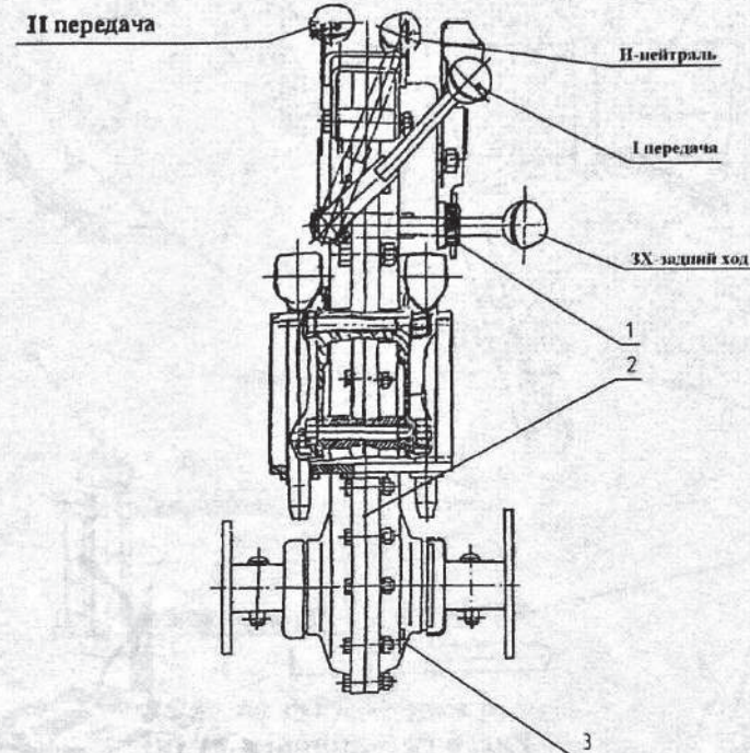
Рис. 5 Редуктор мотоблока
