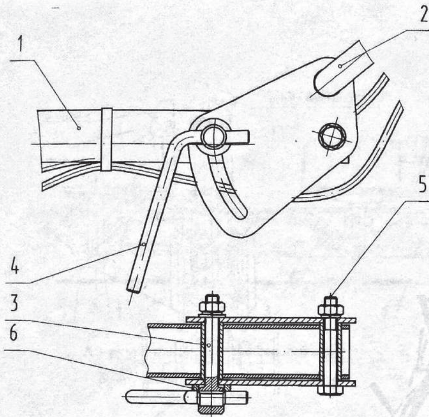
Рис. 6 Регулировка руля
